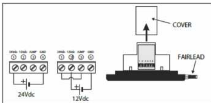
Fig.1 Conexão elétrica
