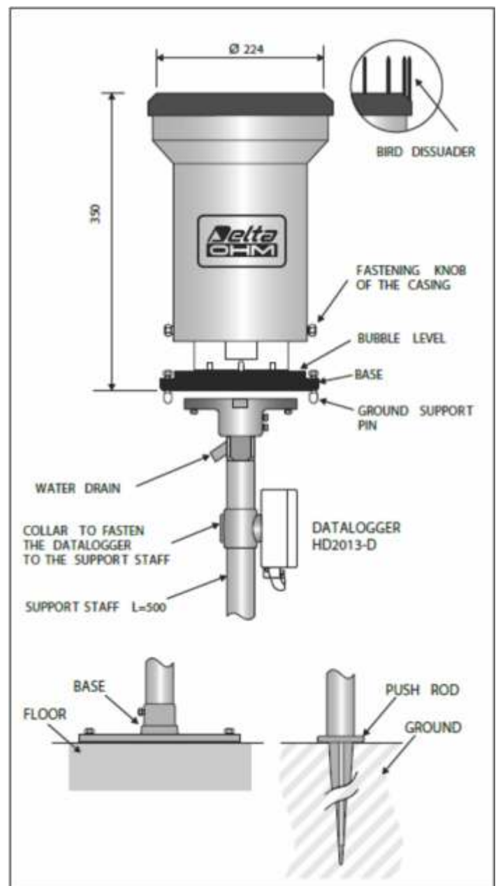
Fig.2 Dimensões e sistemas de fixação no chão e no solo.
